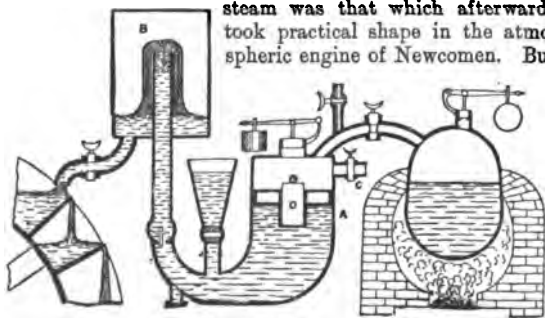
FIG. 3.—Papin, 1705
